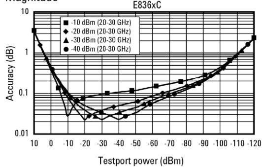
Magnitude
