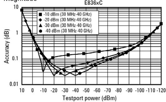
Magnitude
