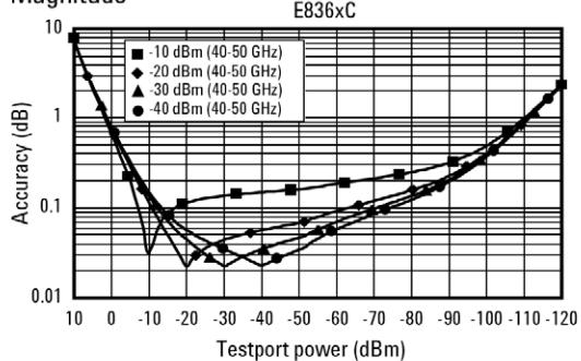
Magnitude
